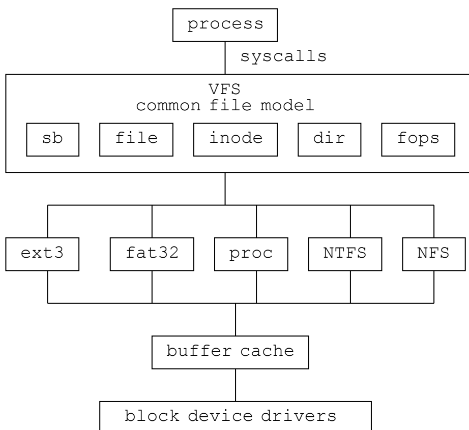
Figura 2: Diseño del virtual file system.
