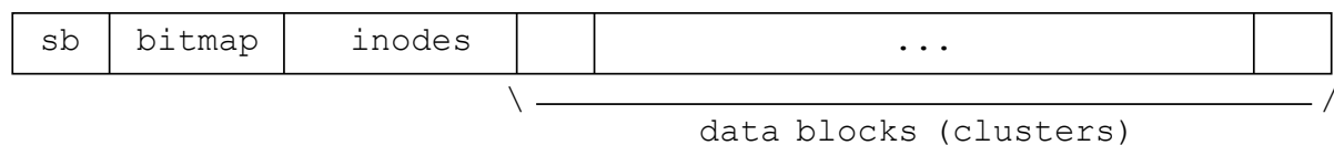
Figura 5: Filesystem con i-nodes.
